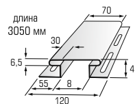
3 соединительная планка
