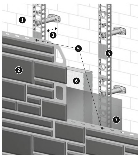
Вариант А: с утеплителем
