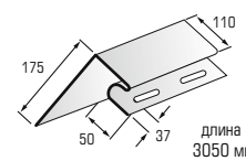
5 околооконная планка
