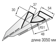
1 внутренний угол
