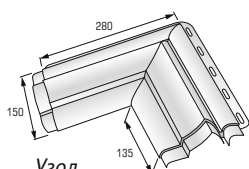
Угол наличника Модерн
