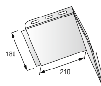
Угол доборного элемента к откосу
