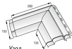
Угол наличника Классик
